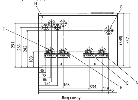
Вид снизу
