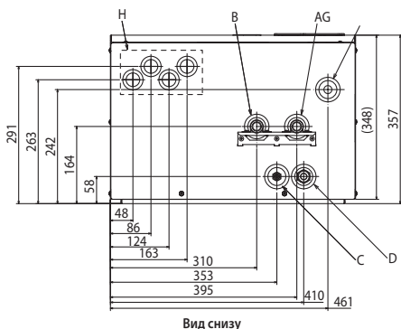
Вид снизу
