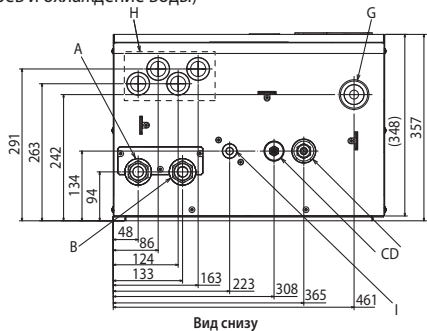
Вид снизу
