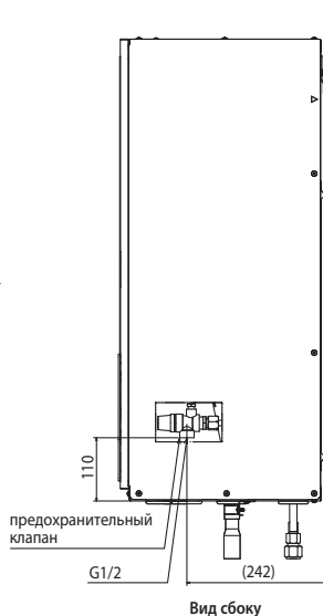
Вид сбоку
